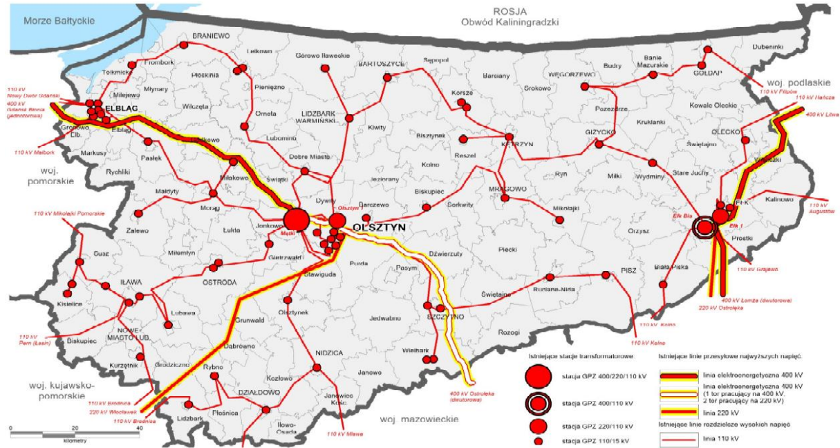
Rysunek 21. Przebieg linii przesyłowych najwyższych napięć w województwie warmińsko-mazurskim
